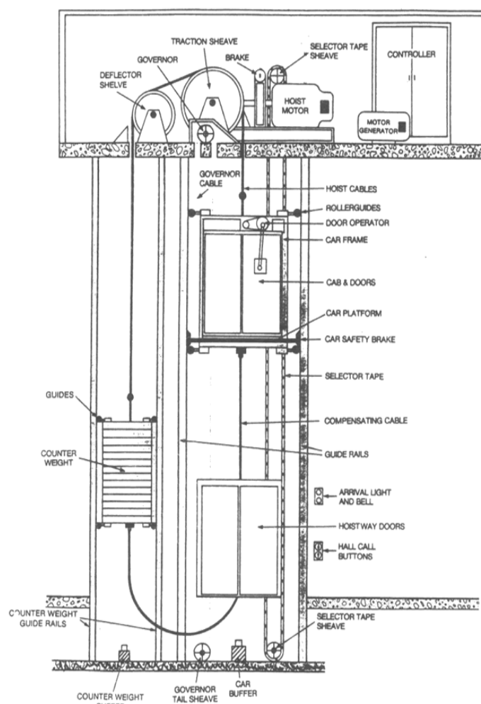
Tractielift met machinekamer
